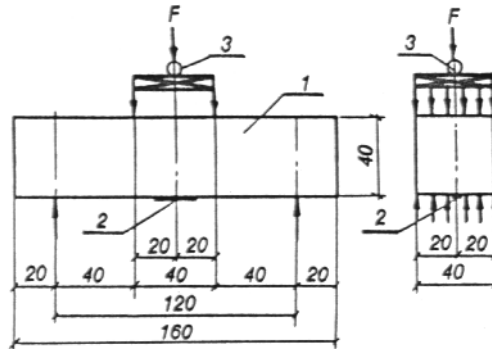
1 — опытный образец; 2 — тензорезистор базой 20 мм; 3 — электрический силоизмеритель
